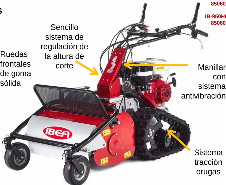
Sistema de corte de martillos flotantes “Y” contra rotura por impactos
